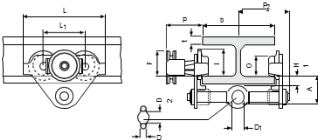
HTG 10 TON
