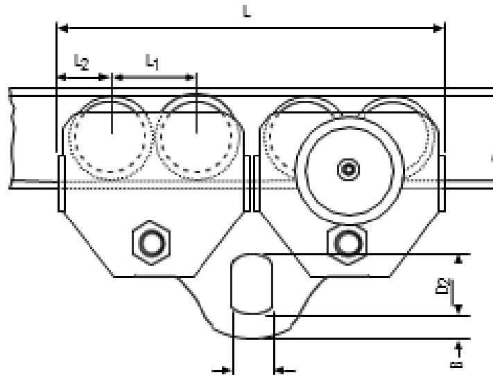
HTG 20 TON
