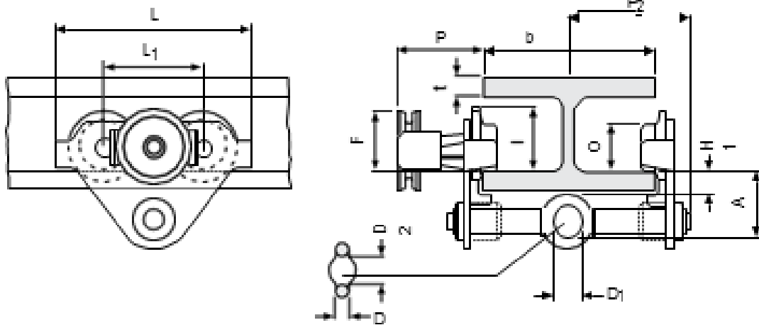
HTG 0.5 – 5 TON
